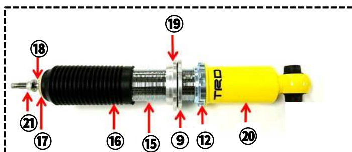
⑭ ショックアブソーバー (リヤ)
