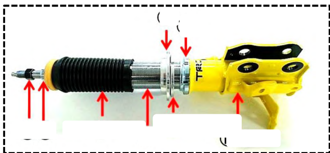
ショックアブソーバー(フロント)
